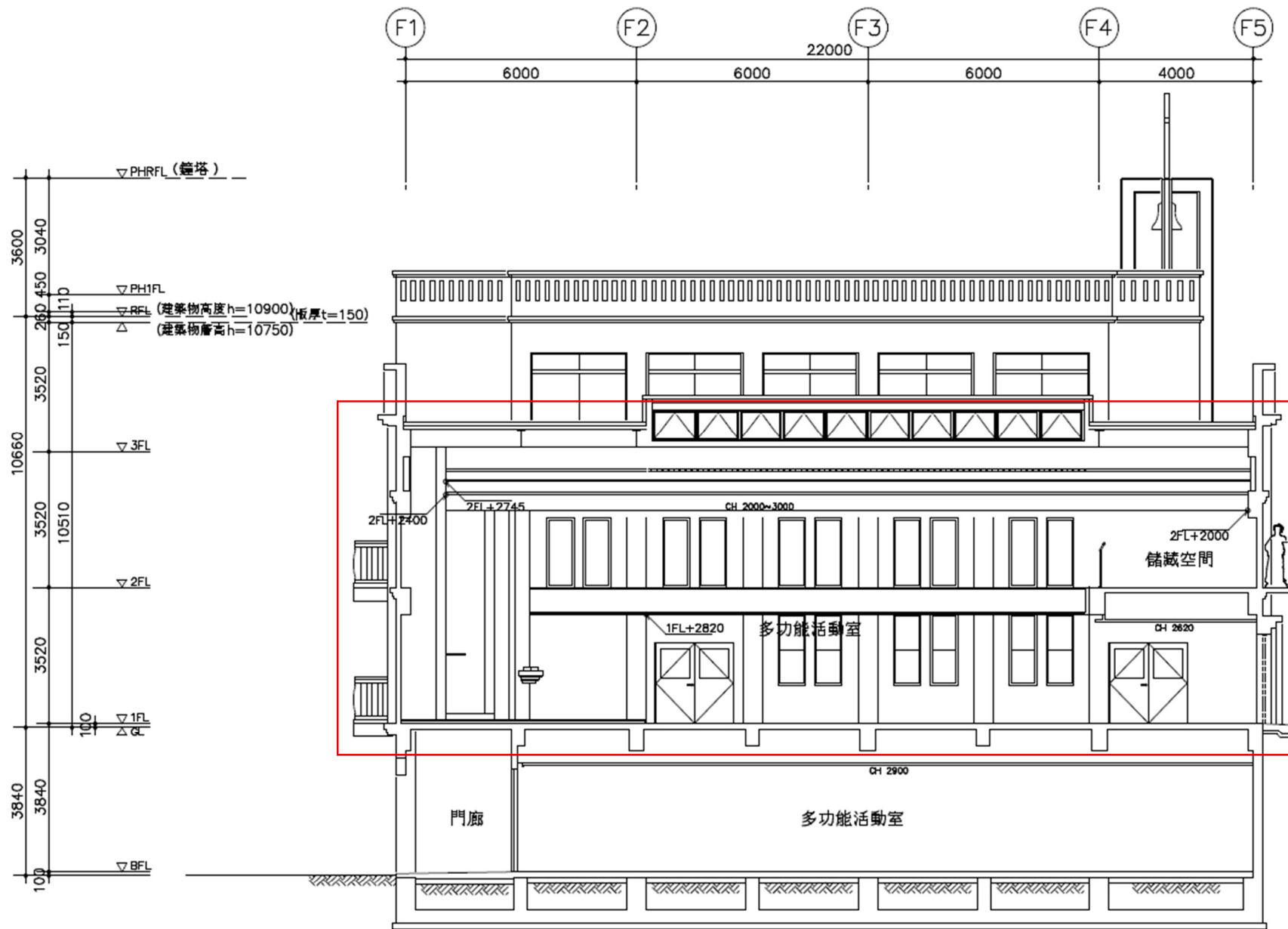
橫向剖面圖 -1
